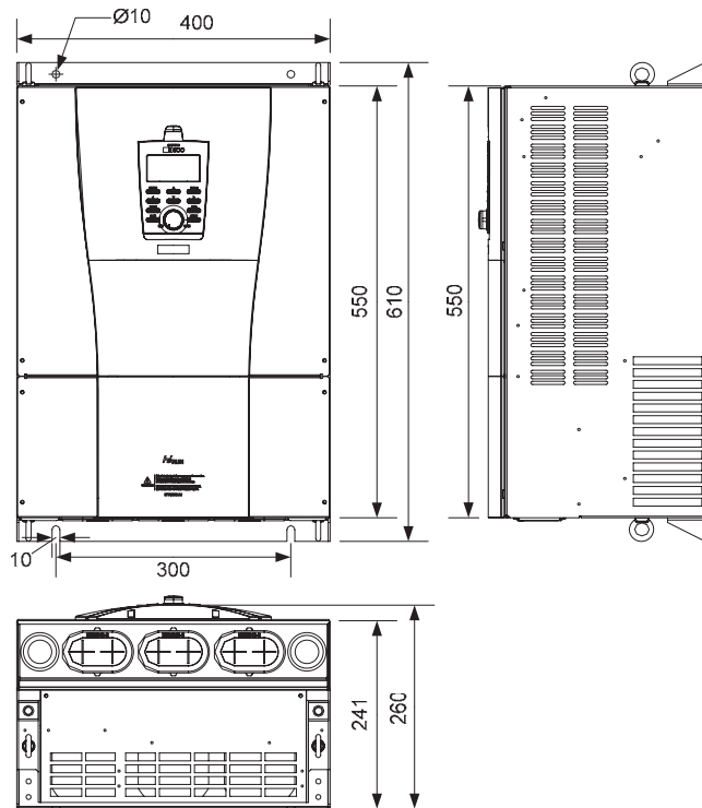
Рис. 16.3 Размеры модели N700-370LF/370HF, N700-450LF/450HF
