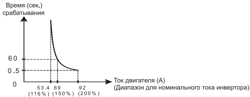
Рис. 8-7 Характеристика регламента времени срабатывания (N700V - 110 LF)
