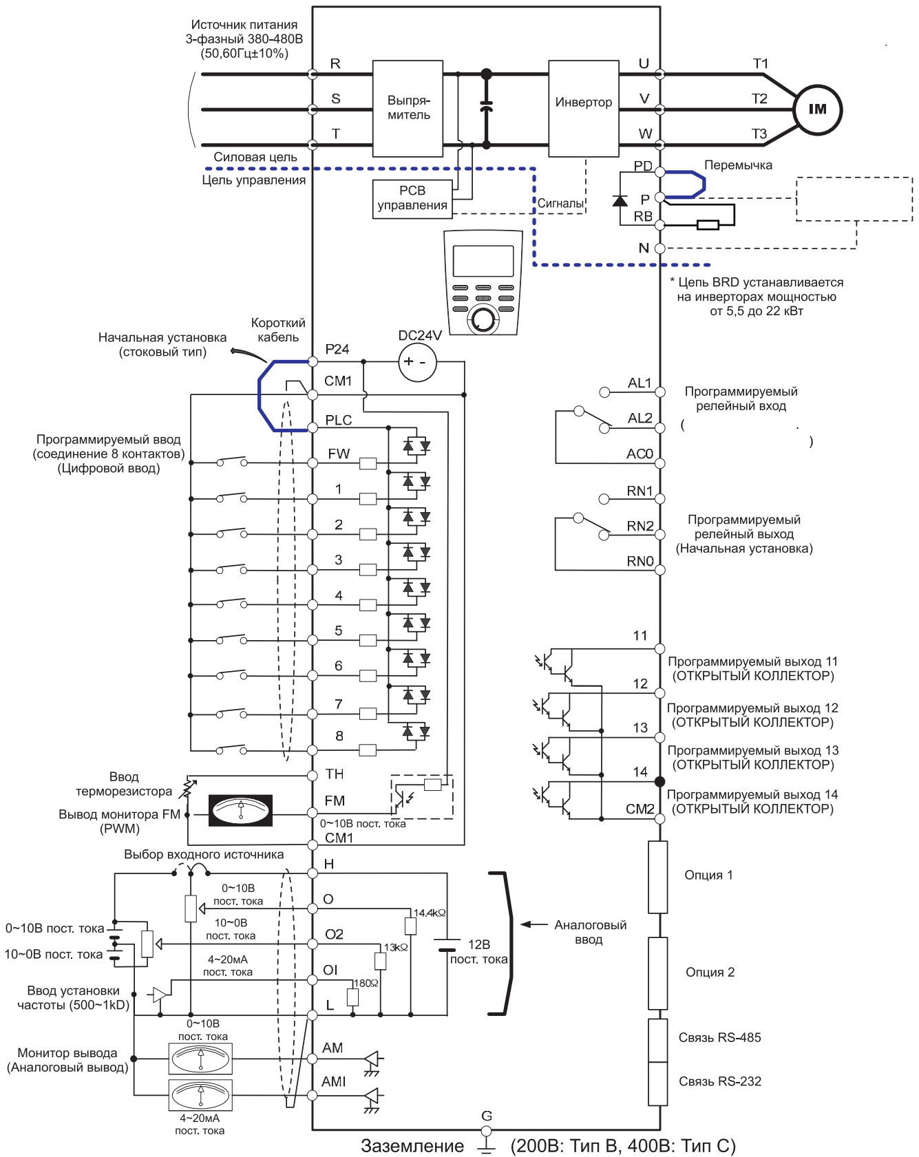
Рис. 2-5 Схема клеммных соединений
